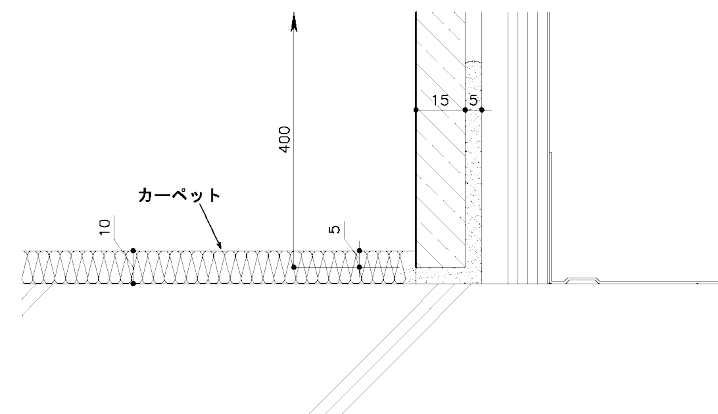
床カーペット取合の床接合図
