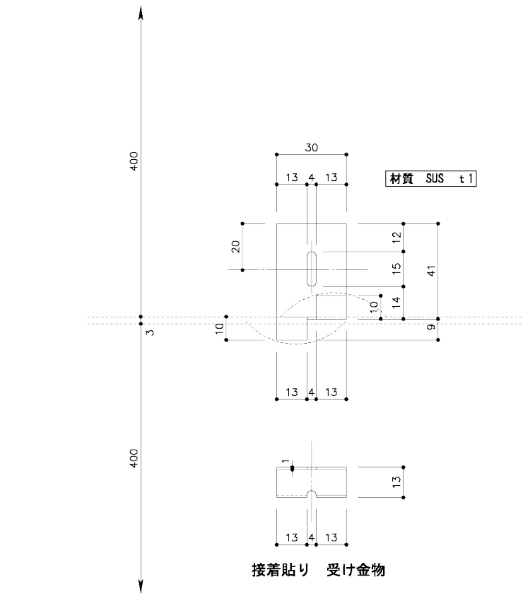
床カーペット取合の床接合図
